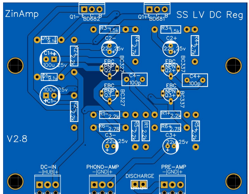
Bare PCB
